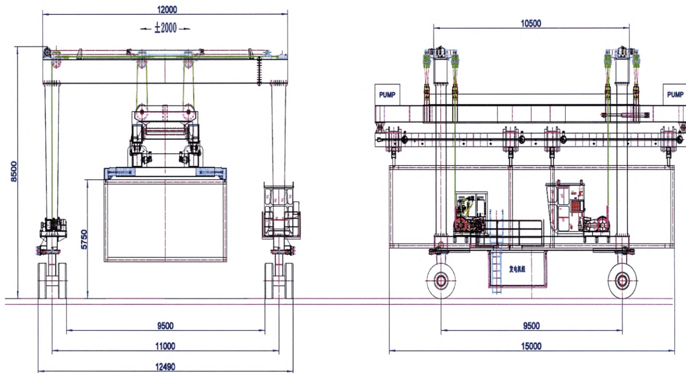
Рисунок 23.8 – Портальные транспортеры
