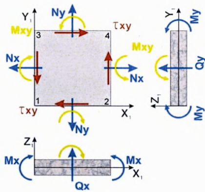
Рисунок 20.2 – Усилия в оболочке
