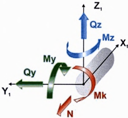
Рисунок 20.1 – Усилия в сечении стержня
