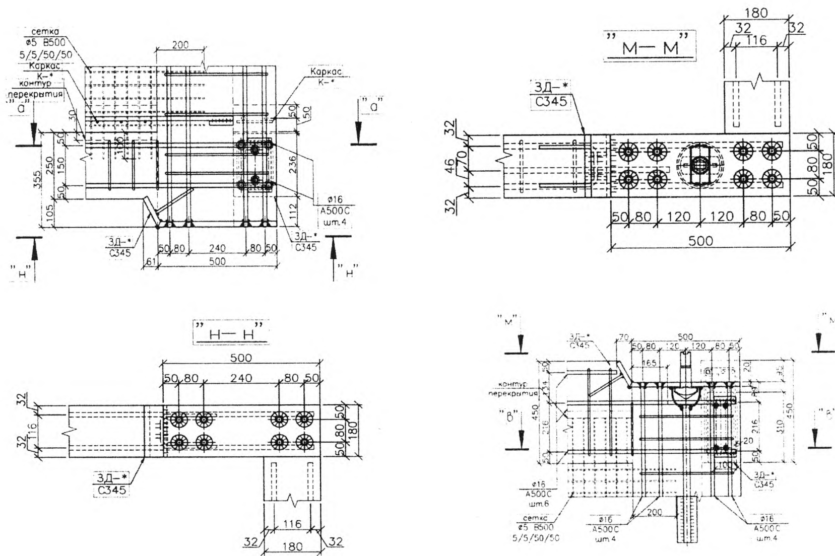
Рисунок 16.7 – Конструктивное решение узлов передачи вертикальных усилий через пилоны и нижние обвязочные балки
