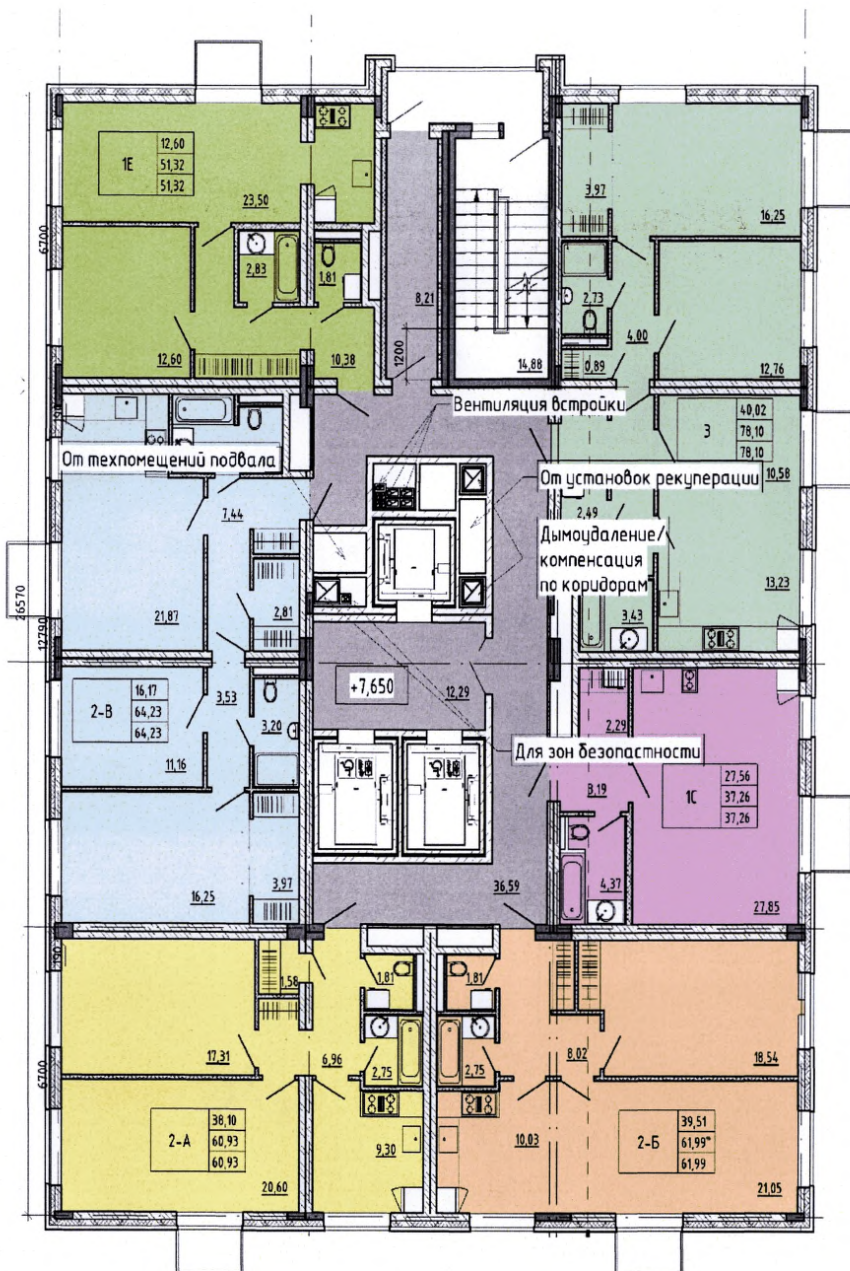
Рисунок 21.3 – Схема размещения на этаже вертикальных инженерных сетей на примере жилого здания система теплоснабжения
