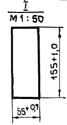
Вырез под крепление РС29
