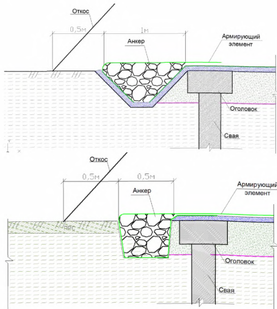
Рисунок 5 – Схемы конструктивных решений по анкеровке армирующего элемента
