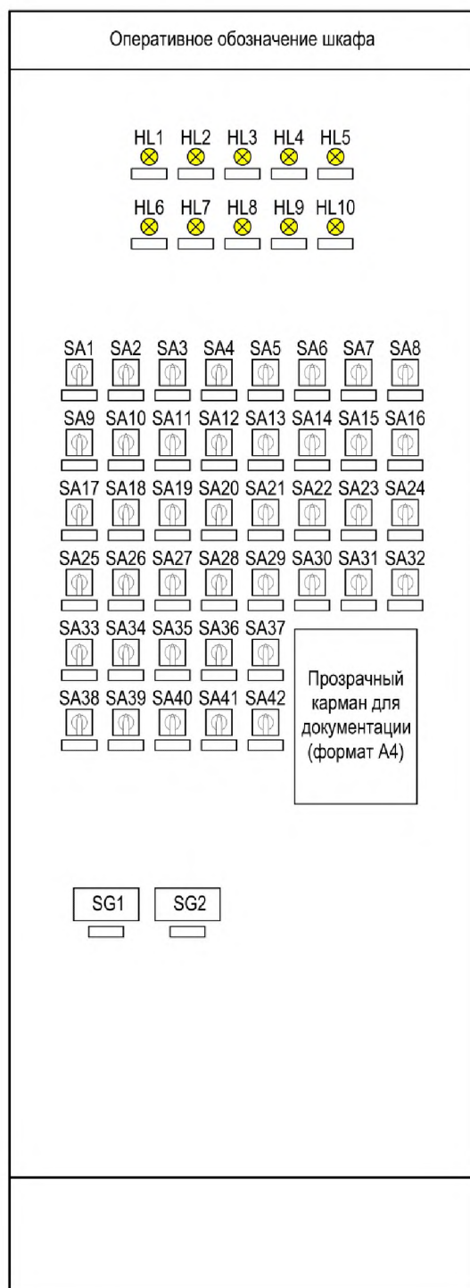
Рисунок 15.2.1 - Эскиз общего вида ШЭТ ОВ
