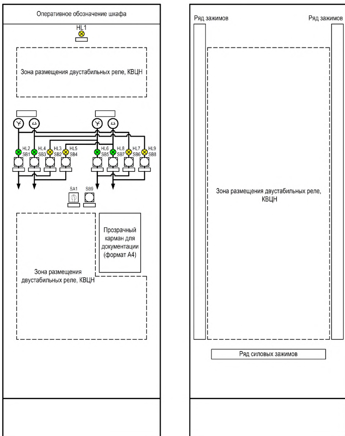
Рисунок 14.5.1 - Эскиз общего вида ШЭТ ЦН.2-1
