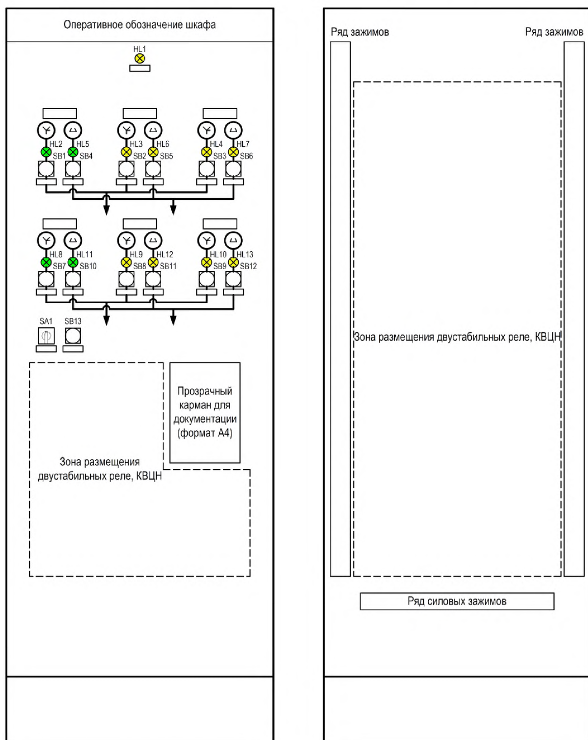
Рисунок 14.6.1 - Эскиз общего вида ШЭТ ЦН.3
