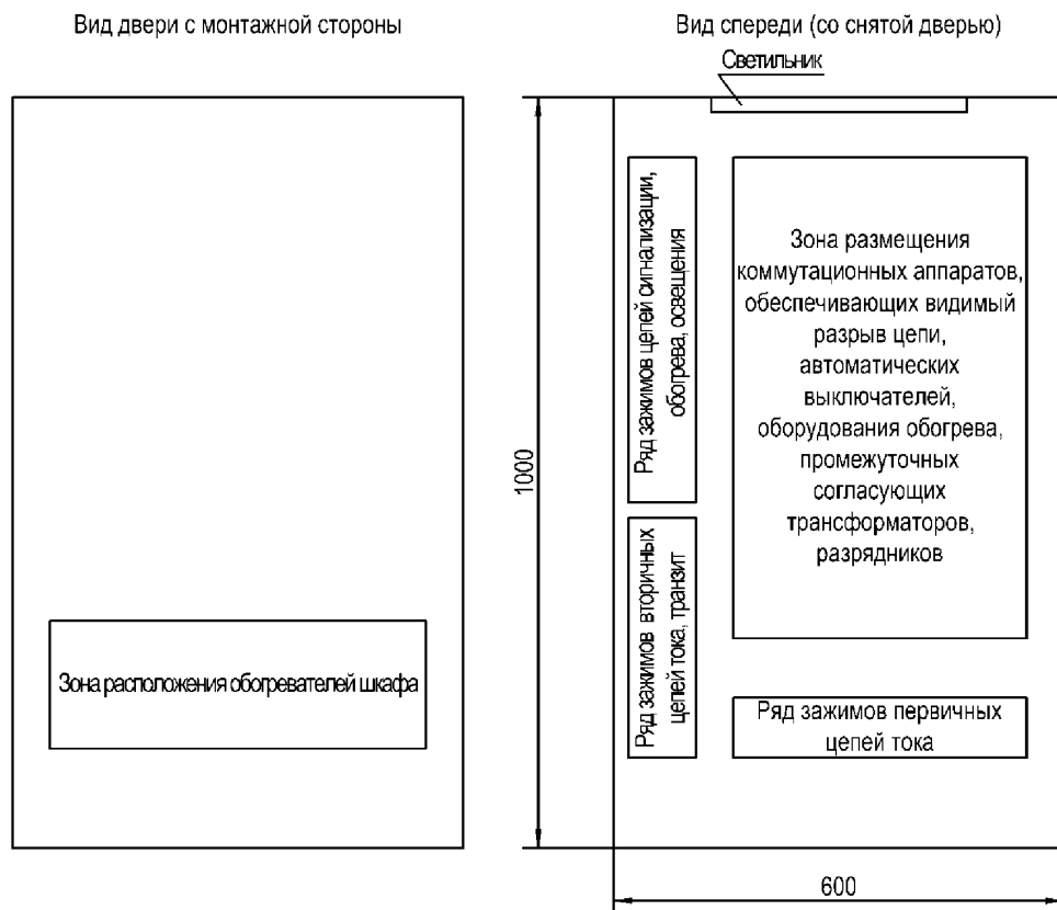
Рисунок 13.3.1 - Эскиз общего вида ШЭТ ТПС.3
