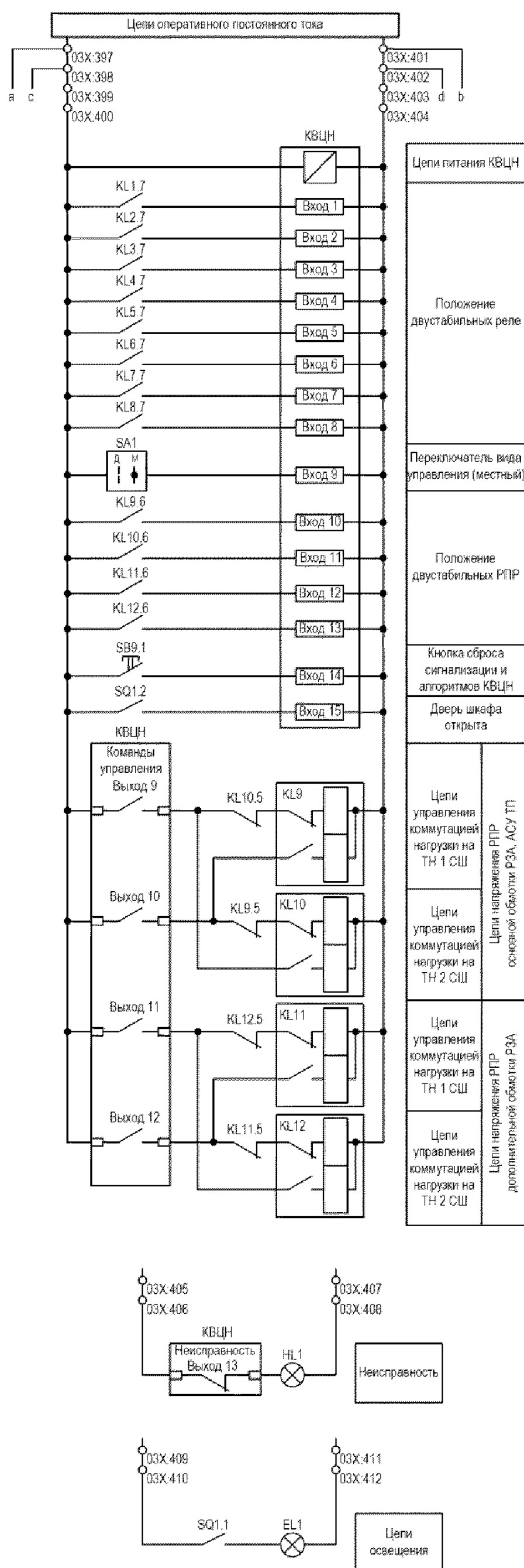
Рисунок 14.5.2 - Схема электрическая принципиальная ШЭТ ЦН.2-1, часть 2
