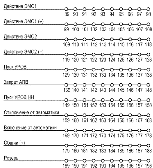
Рисунок 15.2.2 - Схема электрическая принципиальная ШЭТ ОВ, часть 1
