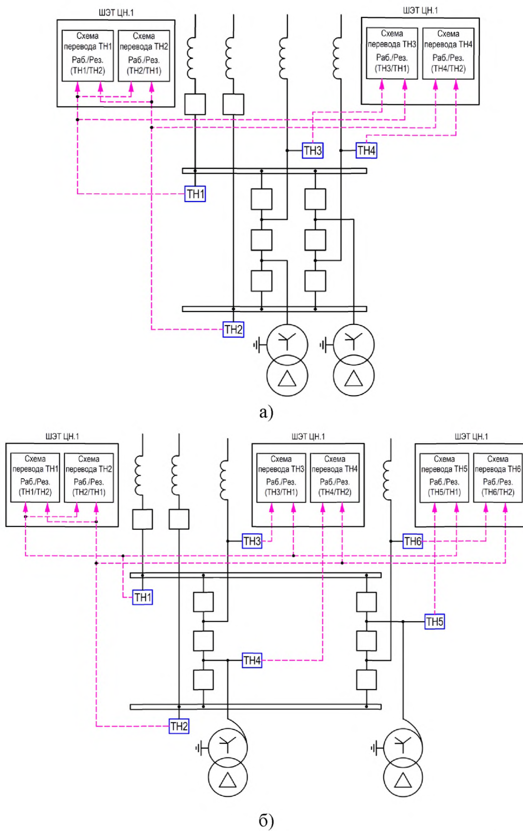
Рисунок А.9 - Поясняющая схема организации ЦН для схем РУ 110-9АН, 220-9АН с трансформатором (а), с автотрансформатором (б)
