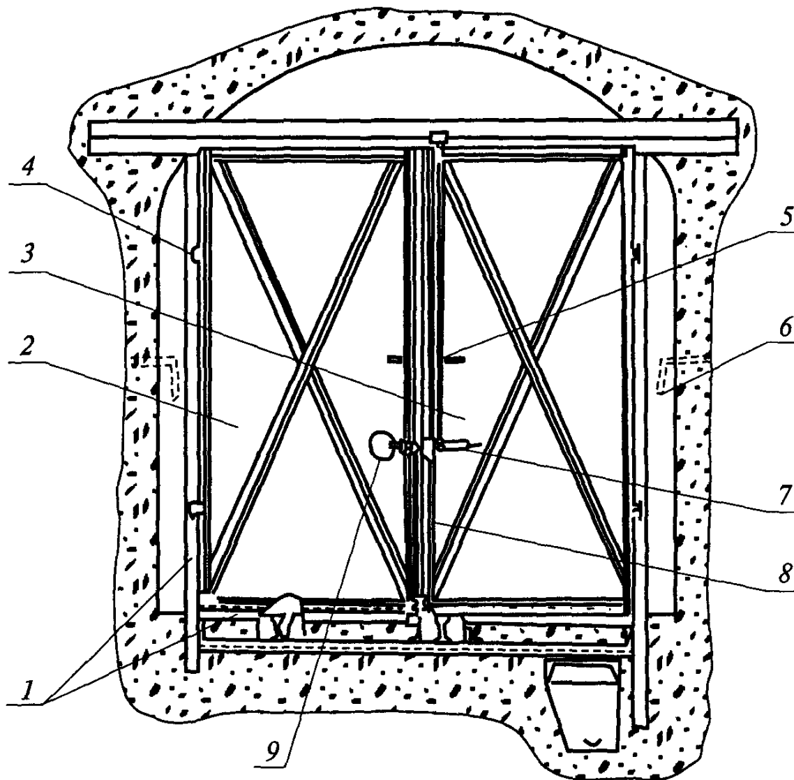
Рис. 6.1. Противопожарная дверь для однопутевой выработки
