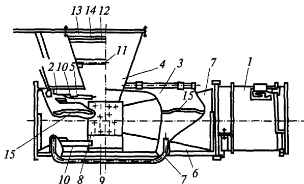
Рис. 8.12. Устройство «Вихрь»:
