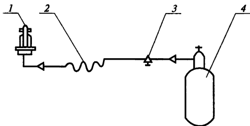
Рис. 8.11. Схема испытания предохранительного клапана: 1 — клапан; 2 — труба; 3 — редуктор; 4 — баллон
