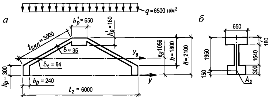
Рисунок 5.7.7 – Приведенные поперечные сечения складки
