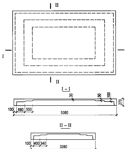
Рисунок 5.8.4 – Геометрия панели
