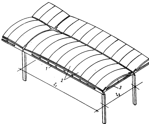
Рисунок 5.3.1 – Длинная цилиндрическая оболочка
