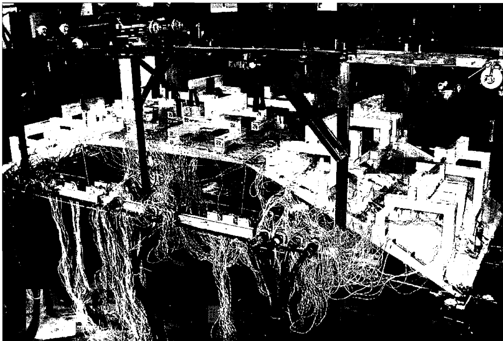
Рисунок 6.1 – Общий вид испытания модели сводчатого покрытия
