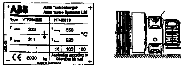
Фирменный шильд турбокомпрессора
