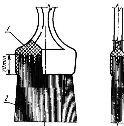
Исполнение флейцевой кисти типа КФ
