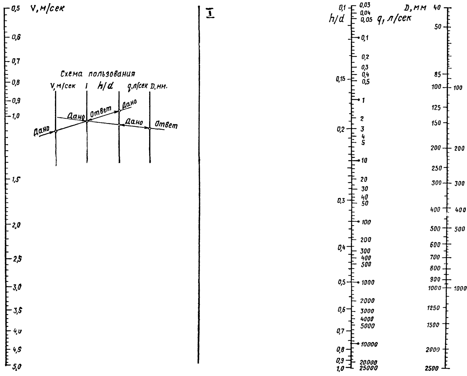
Рис. 2. Номограмма для определения диаметров канализационных трубопроводов
