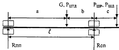
Рис. А.5. Схема нагружения вала якоря тяговых электродвигателей
