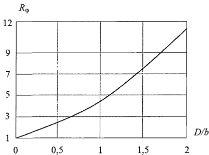
Рисунок 6.1 — Графики определения коэффициентов R_z , R_\phi , R_x для расчета коэффициентов жесткости оснований заглубленных фундаментов»
