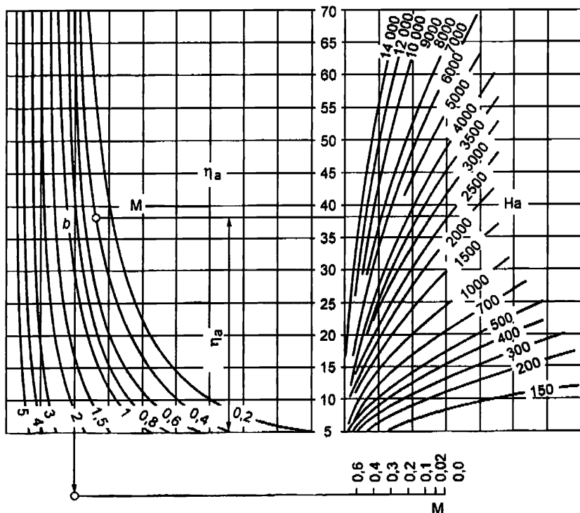
Рисунок Р.1 - Номограмма для расчета радиуса охлаждения и оттаивания
