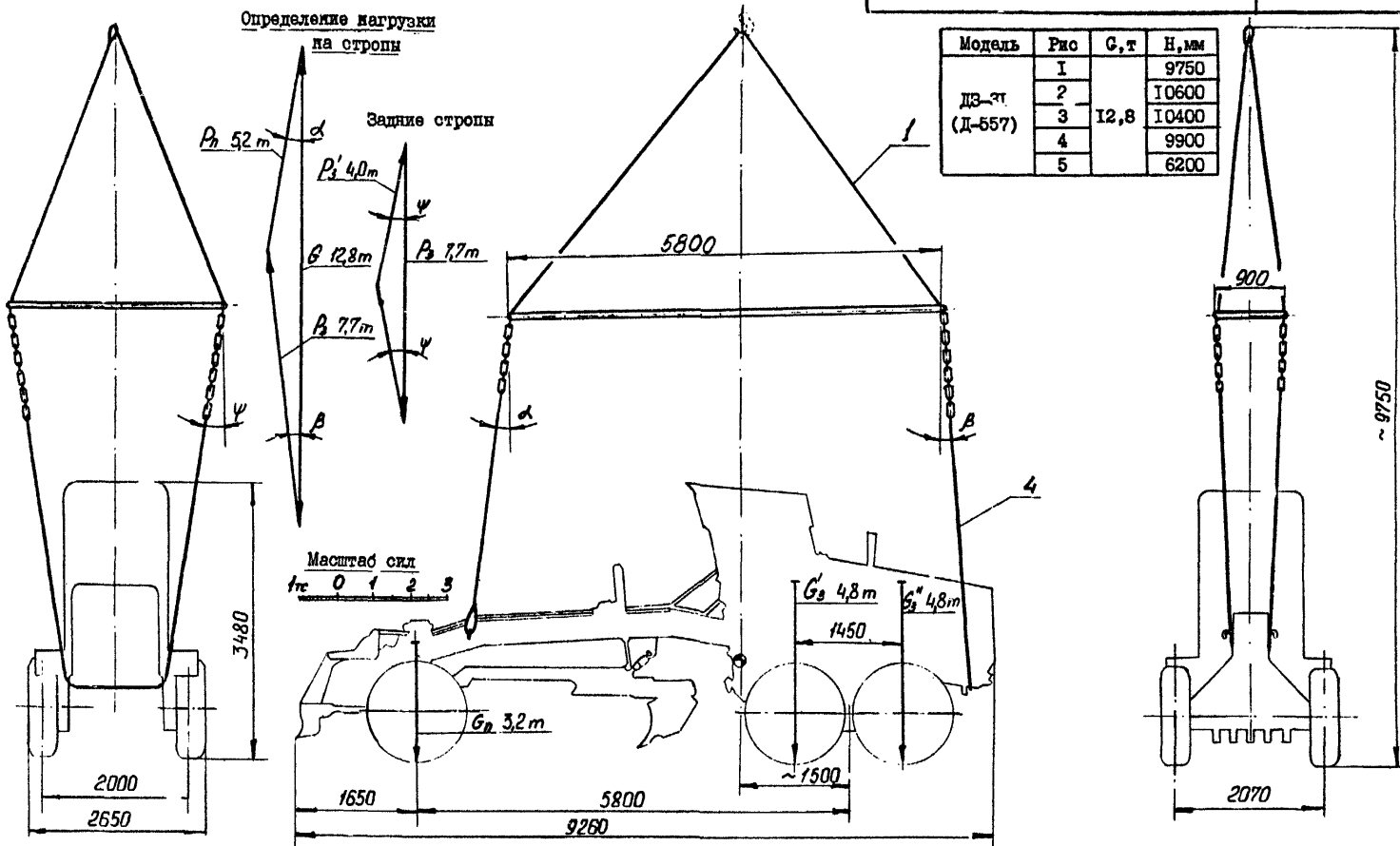
Схема стропки автогрейдера ДЗ-31 ( Д-557 )
