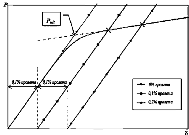
Примечание: P – давление на перекрытие; \delta – максимальная стрелка прогиба рамного шпангоута или несущего стрингера
