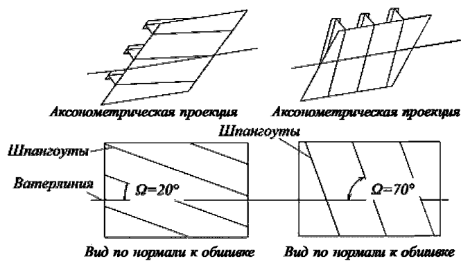
Рис. 1.2.4.2 Угол наклона \Omega набора наружной обшивки
