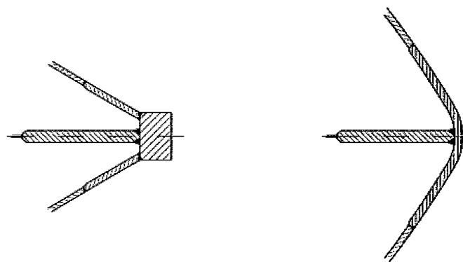
Рис. 10.5.7.1 Примеры допустимой конструкции форштевня
