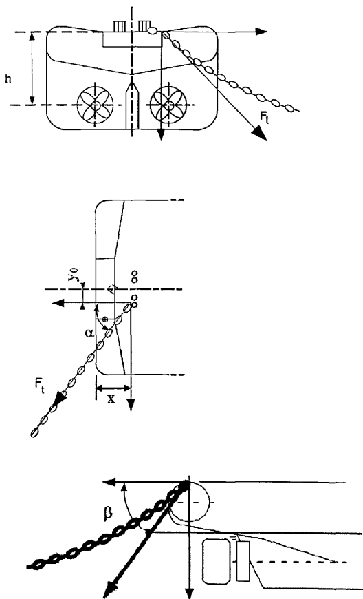
Рис. 1.1.1 Схема расположения углов \alpha и \beta и расстояний h , x и y . Вектором F_t обозначено направление действия силы натяжения троса
