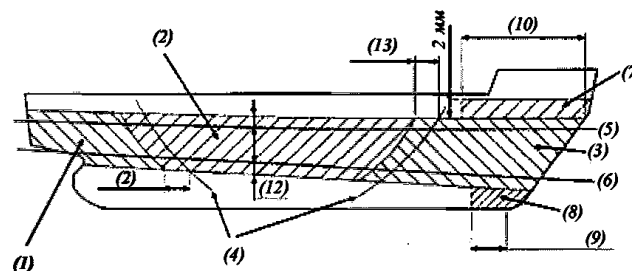
Рис. 10.5.1.1 Районы ледовых усилений корпуса судна:
