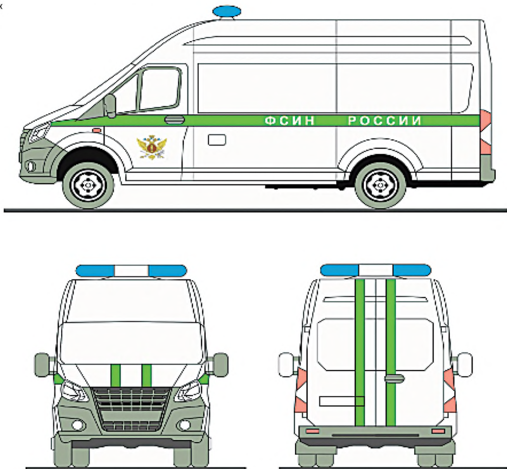
Рисунок А.68 — Цветографические схемы автомобилей уголовно-исполнительной системы Российской Федерации
