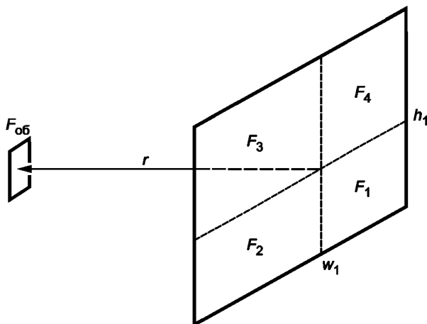
Рисунок А.3.2. Облучаемый материал F_{\text{об}} расположен напротив середины поверхности пламени F_{1-4} , где w_1 и h_1 — длина и высота соответствующей части поверхности пламени.
