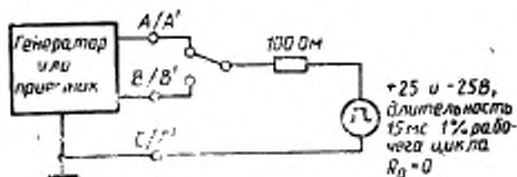
Рис. 15 Проверка переходного напряжения
