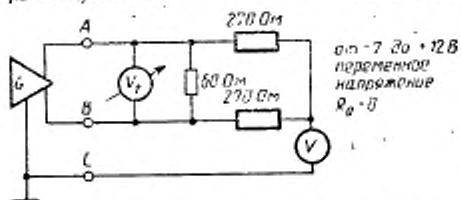
Рисунок 9 Измерение напряжения нагруженного выхода
