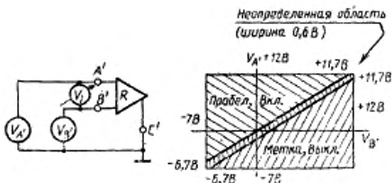
Рисунок 11 Диапазон входных напряжений
