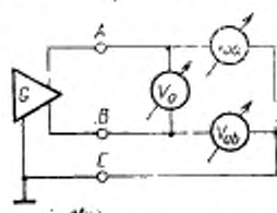
Рисунок 7 Измерение напряжения разомкнутой цепи
