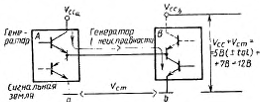
Рисунок 16. Соперничество генераторов с одним генератором-источником
