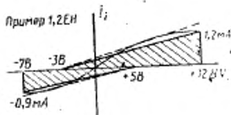
Рисунок 6 Определение значения ЕН
