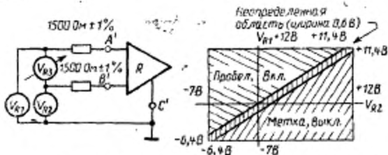
Рисунок 12 Измерение рассогласования на входе
