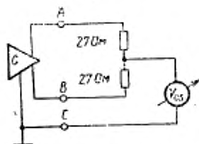
Рисунок 8 Измерение смещения напряжения
