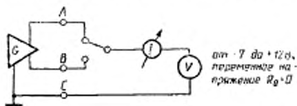
Рисунок 14 Проверка соперничества генераторов
