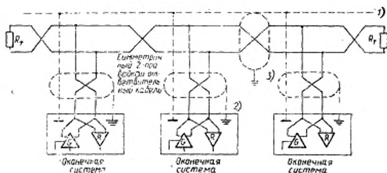
Рисунок 2 Двухпроводная многопунктовая конфигурация
