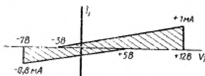
Рисунок 4 Ограничения тока 1,0 ЕН
