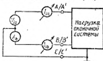
Рисунок 5 Измерение входного тока/напряжения
