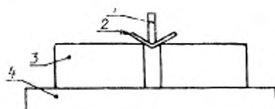
1 — брусок проникающий; 2 — испытываемый образец; 3 — опорная площадка; 4 — устройство для измерения усилия
