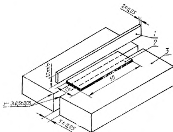
1 — брусок проникающий, 2 — образец, 3 — опорная площадка
