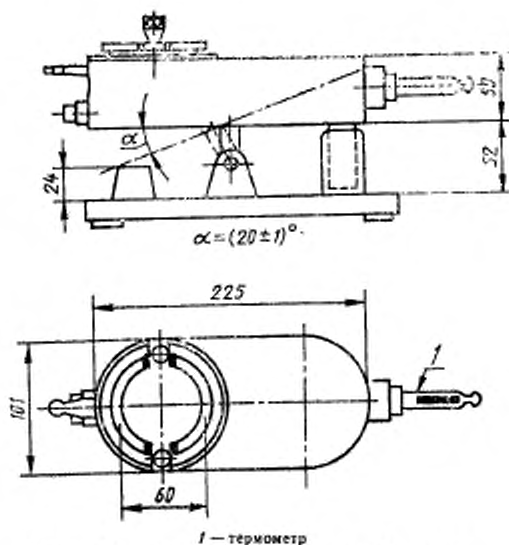
Рисунок 6 — Стандартный пенетrometer Вильямса
