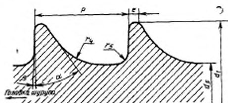
Рисунок 2 — Мелкая резьба (НА)
