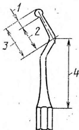
1 — режущая кромка; 2 — шейка; 3 — рабочая часть; 4 — хвостовик
