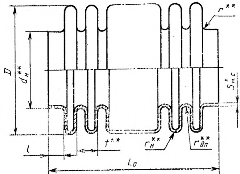
Рисунок 2 — Сильфон, тип 2
