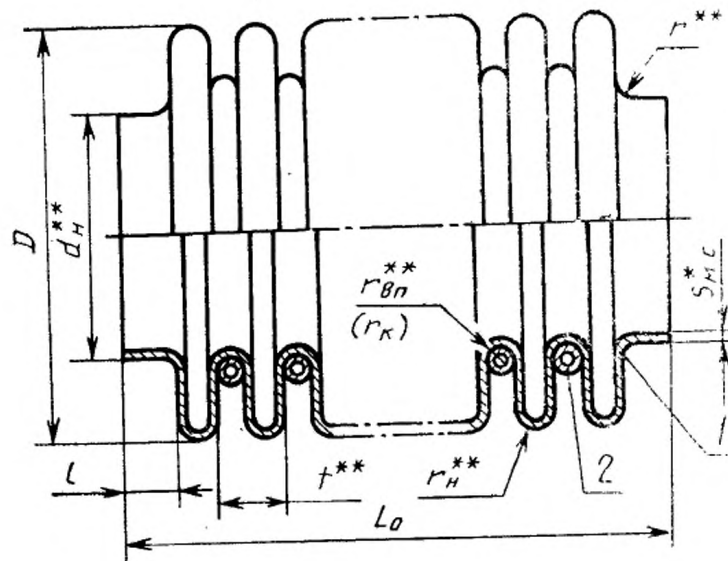
Рисунок 3 — Сильфон, тип 3
