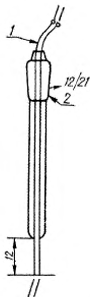
Платиновые электроды: 1 — медные проволочки, одна из которых изолирована пластмассовой оболочкой; 2 — коническое соединение из стекла, стандарт 12/21
