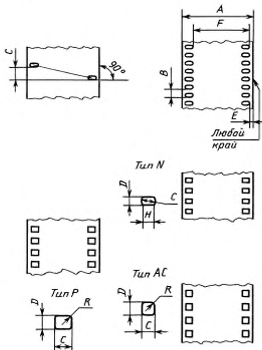
Типы перфораций
