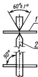
1 — калибровочная проволока; 2 — твердосплавный резец
