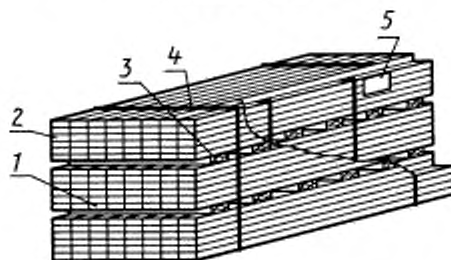
1 — деталь короткая; 2 — деталь длинная; 3 — прокладка; 4 — обвязка; 5 — ярлык
