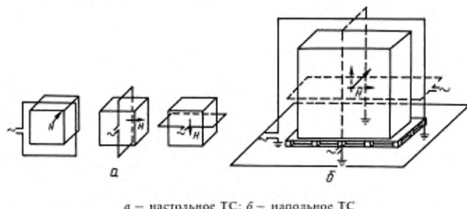
Рисунок 1 — Схема воздействия МППЧ на ТС с использованием иммерсионного метода
