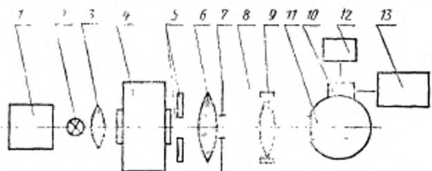
1 — стабилизатор напряжения; 2 — лампа накаливания; 3 — конденсор; 4 — монохроматор (или интерференционный светофильтр); 5 — светофильтр для устранения влияния вредного рассеянного света; 6 — коллиматор; 7 — диафрагма; 8 — объективодержатель; 9 — испытуемый объект; 10 — фотоумножитель; 11 — фотометрический шар; 12 — измерительный прибор; 13 — высоковольтный стабилизатор напряжения
