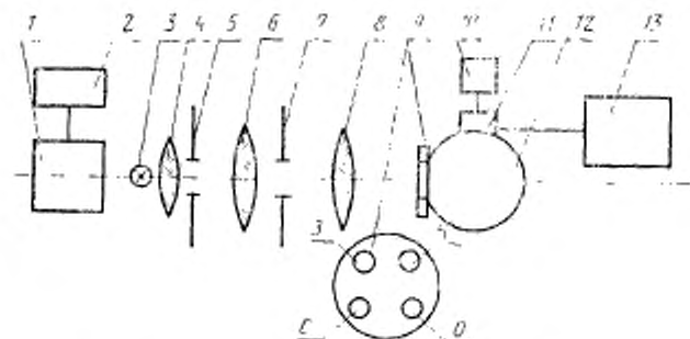
1 — стабилизатор напряжения; 2 — контрольный вольтметр (амперметр); 3 — лампа накаливания; 4 — конденсор; 5 — диафрагма; 6 — коллиматор; 7 — диафрагма; 8 — испытуемый объект; 9 — турель с корректирующими светофильтрами; 10 — измерительный прибор; 11 — фотоприемник; 12 — фотометрический шар; 13 — высоковольтный стабилизатор напряжения
