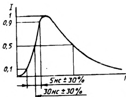
Рисунок Г.2 — Форма волны
