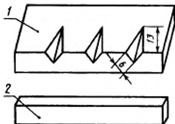
1 — форма для изготовления образцов зола, 2 — вертел (формирующая) пластинка к форме
