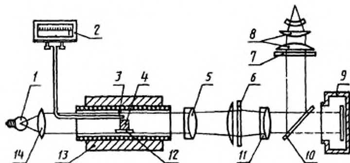
1 — осветитель, 2 — жидкостный термометр, 3 — термонора, 4 — образец из золы, 5 — координатная сетка, 6 — матовое стекло, 7 — линза, 8 — линза, 9 — фотографическая камера, 10 — зеркало, 11 — окуляр, 12 — подставка, 13 — электропривод, 14 — конденсор
