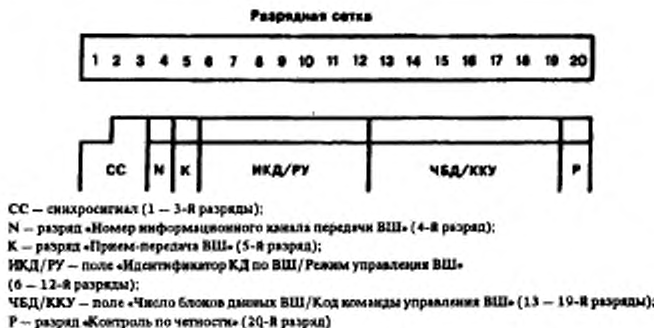
Рисунок 5 — Формат КСВШ
