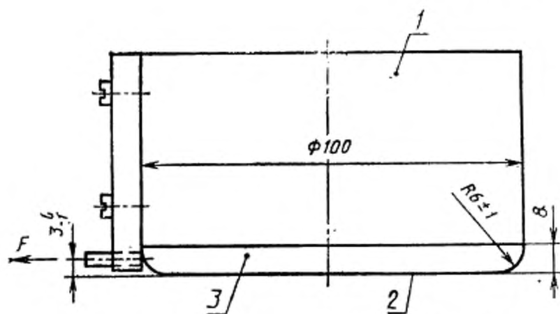
1 — фрикционный цилиндр; 2 — трущаяся поверхность; 3 — диск
