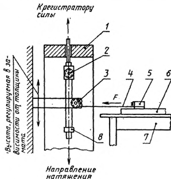
1 — испытательное устройство; 2 — блок крепления к индикатору силы; 3 — блок отклонения; 4 — стальной трос; 5 — фрикционный цилиндр; 6 — мат для прыжков; 7 — опорный стол; 8 — зажимное устройство для крепления троса
