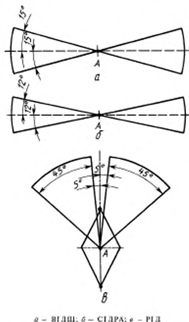
Рисунок Д.1 — Расположение секторов наибольшего значения вертикальной составляющей напряженности поля антенн разных типов
