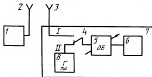
1 — контролируемый радиопередатчик; 2 — антенно-фидерная система; 3 — измерительная антенна; 4 — коаксиальный переключатель; 5 — аттенуатор; 6 — измерительный приемник; 7 — экранированная камера (используется при необходимости); 8 — измерительный генератор
