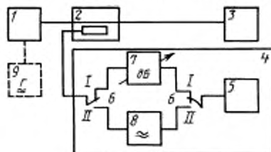
1 – контролируемый радиопередатчик; 2 – направленный ответвитель; 3 – эквивалентное нагрузочное сопротивление или штатная антенна радиопередатчика; 4 – экранированная камера (используется при необходимости); 5 – измерительный приемник; 6 – высокочастотный переключатель; 7 – измерительный аттенуатор; 8 – фильтр; 9 – генератор сигналов низкочастотный
