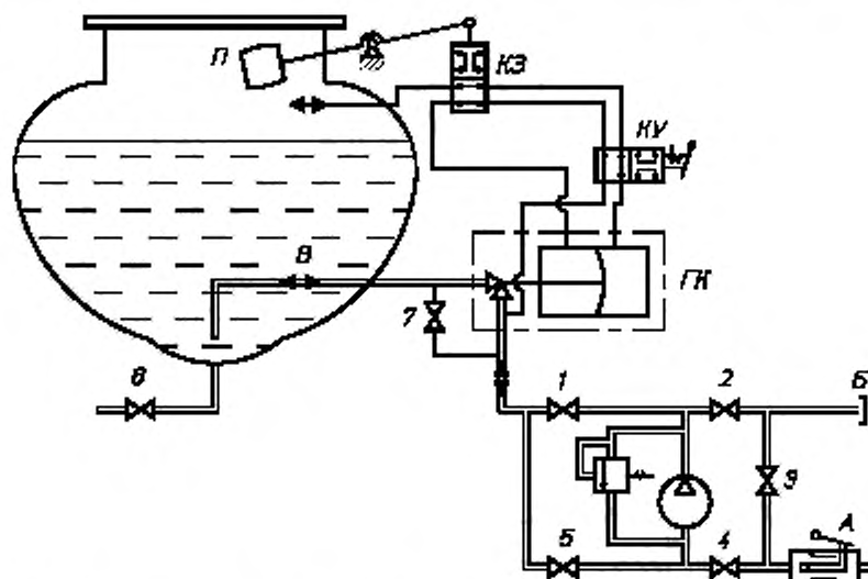
Рисунок Д.1 — Унифицированная принципиальная технологическая схема автоцистерны
