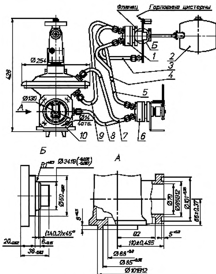
1 — кран золотниковый, 2 — поплавок, 3, 4, 5, 7, 8, 9 — соединительные магистрали; 6 — клапан управления; 10 — гидроклапан
