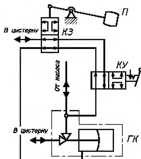
Рисунок А.1 — Схема гидравлическая принципиальная ограничителя наполнения
