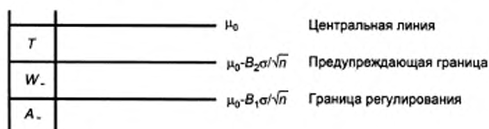
Рисунок 3 — Зоны качества для статистического управления с односторонним критерием — нижние границы
