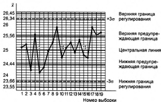
Рисунок Б.1 — Пример контрольной карты для арифметического среднего с предупреждающими границами
