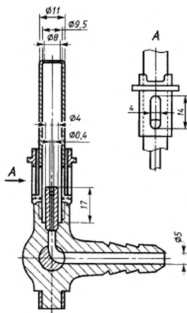
Рисунок 1 — Горелка
