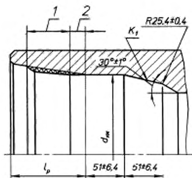
1 — длина резьбы с полным профилем; 2 — длина резьбы со срезанными вершинами
