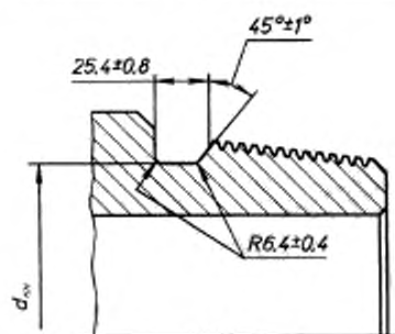
Рисунок В.1 — Разгрузочная канавка ниппеля
