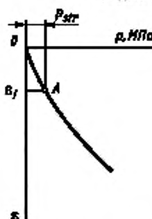
График 2 — Относительное сжатие глинистого грунта при частичном разуплот- нении в зависимости от давления p
