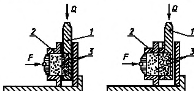
1 — подвижная часть прибора (срезная каретка); 2 — неподвижная часть прибора (корпус); 3 — образец; Q — касательная нагрузка; F — нормальная нагрузка
