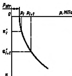
График 1 — Относительное сжатие водонасыщенного грунта в зависимости от давления p
