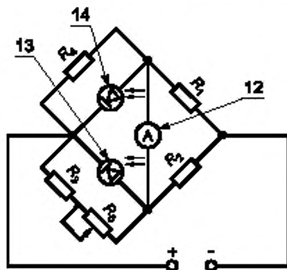
12 — регистрирующее устройство; 13, 14 — приемник.
