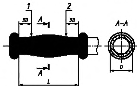
L — длина; B — ширина; l — задняя контрольная точка рукоятки; 2 — передняя контрольная точка рукоятки
