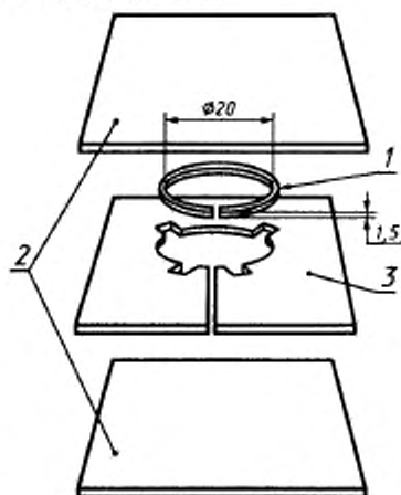
1 — разъемное кольцо; 2 — покрывные пластины; 3 — фиксирующая пластина
