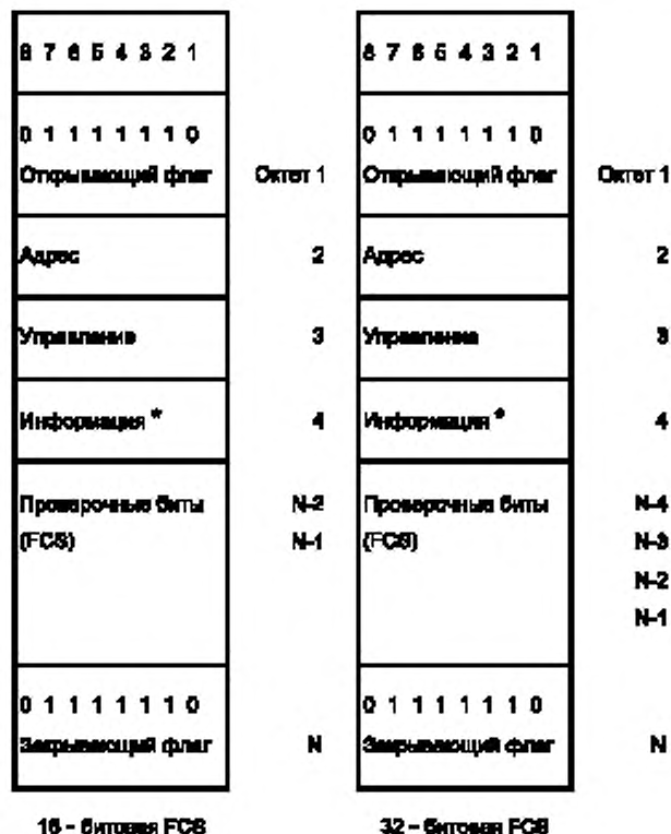
Рисунок 2 — Структура кадра
