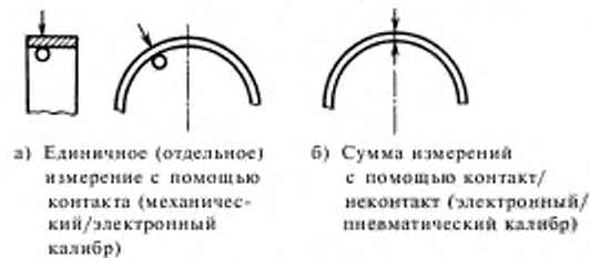
Рисунок 2 — Принцип измерения толщины стенки
