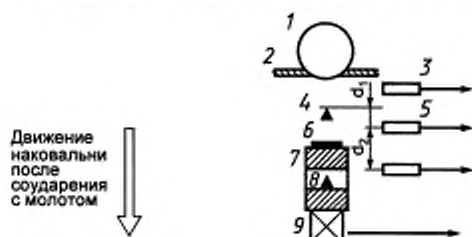
1 — молот; 2 — улавливающее устройство; 3 — фотодатчик запуска; 4 — нож в состоянии покоя; 5 — фотодатчик системы измерения скорости; 6 — прокладка; 7 — наковальня; 8 — светоотсекающий нож; 9 — калибруемый акселерометр
