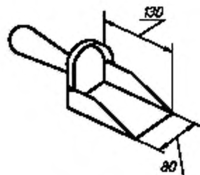
Рисунок 2 — Совок
