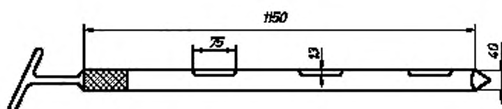
Рисунок 4 — Цилиндрический пробоотборник (секционный для отбора проб из насыпи)
