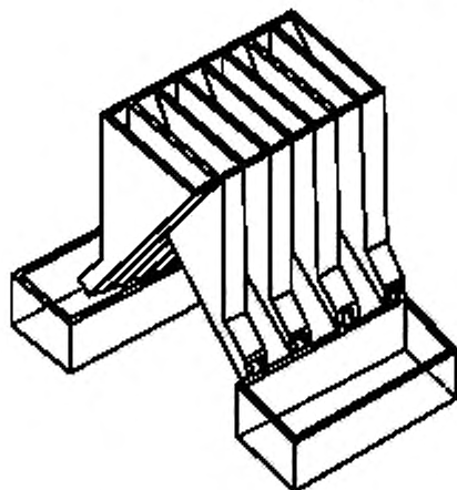
Рисунок 9 — Многожелобковый делитель
