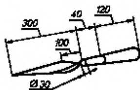
Рисунок 1 — Щуп открытого типа
