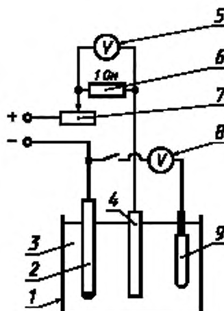
1 — емкость; 2 — испытуемый образец; 3 — электролит; 4 — инертный анод; 5 и 8 — вольметры; 6 — эталонное сопротивление; 7 — реостат; 9 — электрод сравнения
