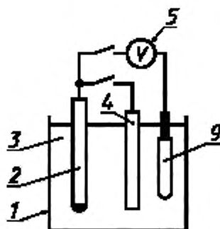
1 — емкость; 2 — испытуемый образец; 3 — электролит; 4 — магний; 5 — вольметр; 9 — электрод сравнения
