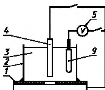
1 — пластина (карта) — испытуемый образец; 2 — труба из полиэтилена; 3 — электролит; 4 — магний; 5 — вольметр; 9 — электрод сравнения
