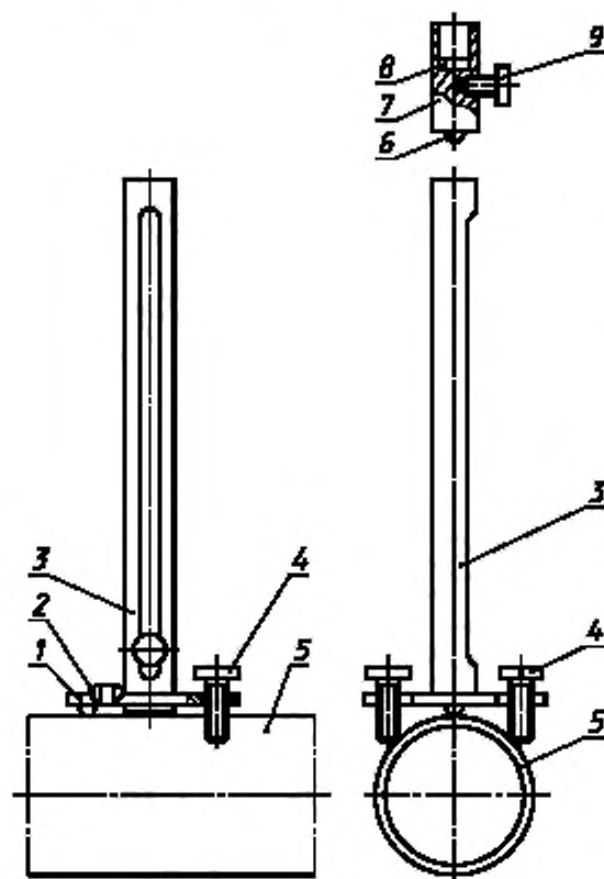
1 — основание; 2 — уровень (индикатор горизонтальности); 3 — направляющая; 4 — винты-ножки; 5 — труба с испытуемым покрытием; 6 — стальной боек; 7 — груз; 8 — утяжелитель; 9 — винт-рукоятка
