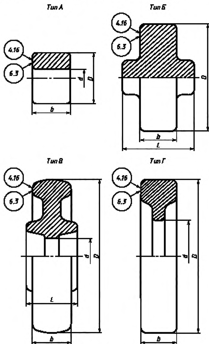
Рисунок 1 — Типы заготовок
