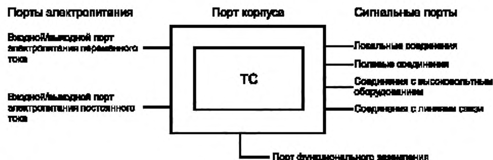
Рисунок 1 — Порты ТС
