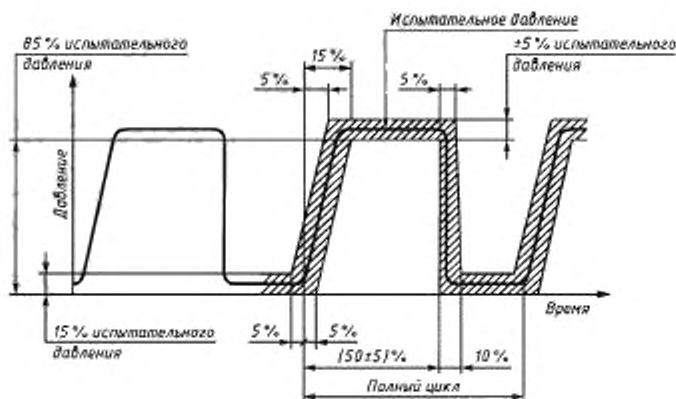
Рисунок 8 — Циклограмма изменения давления в испытываемом трубопроводе
