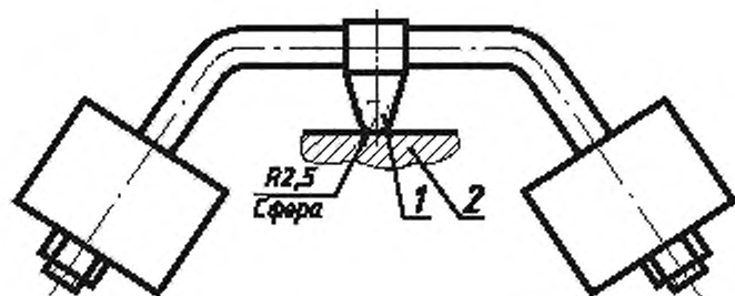
Рисунок 18 — Аппарат для испытания давлением шарика (9.14.2)
