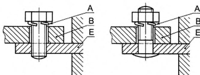
Рисунок 1С.3 — Примеры пластинчатых выводов
