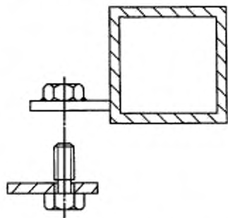
Рисунок 11 — Пример нетеряющихся средств крепления
