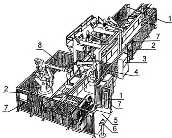
1 — фотоэлектрический барьер; 2 — съемное защитное устройство с блокировкой; 3 — коммутационный шкаф; 4 — внутреннее ограждение, разрешающее доступ в определенном месте; 5 — изолирующий коврик; 6 — устройство для двуручного включения; 7 — орган возврата в исходное положение; 8 — съемное защитное устройство
