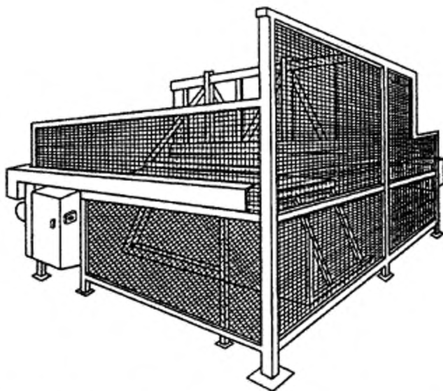
Рисунок 2 — Пример съемного дистанционного защитного устройства
