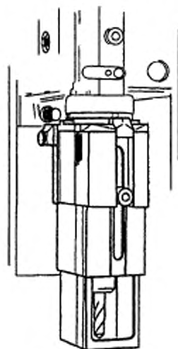
Рисунок 5 — Регулируемое съемное защитное устройство
